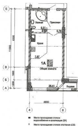
Фрагмент плана 2-5-го этажей. 1-но комнатная квартира 1А
